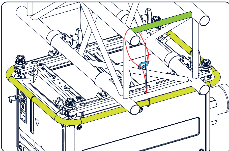
Изображение 3-55 Страховочные тросы
