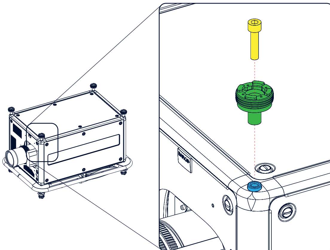
Изображение Е-1 Установка узлов штабелирования
