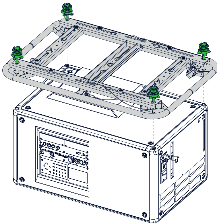
Изображение 3-46 Установка рукоятки для переноски
