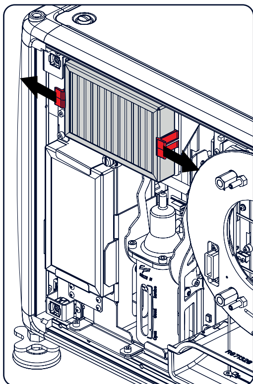
Изображение 16-12 Замена фильтра
