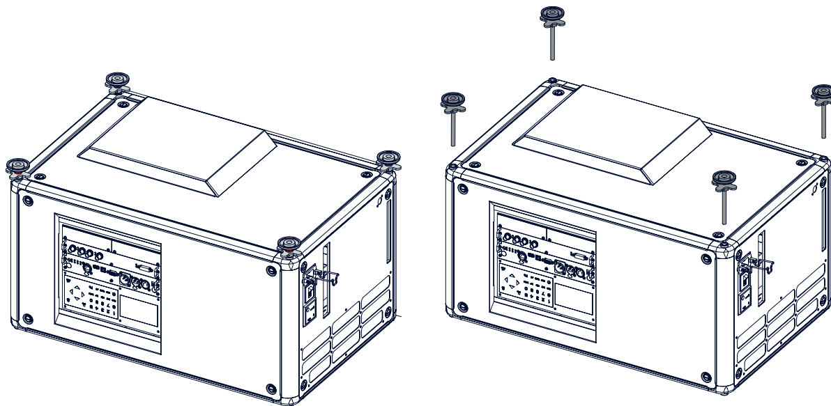
Изображение 3-45 Снятие ножек
