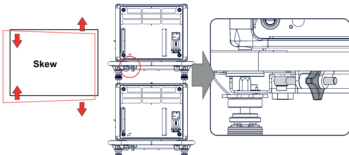
Изображение Е-8 Регулировка смещение оси по горизонтали в установленных друг на друга проекторах
