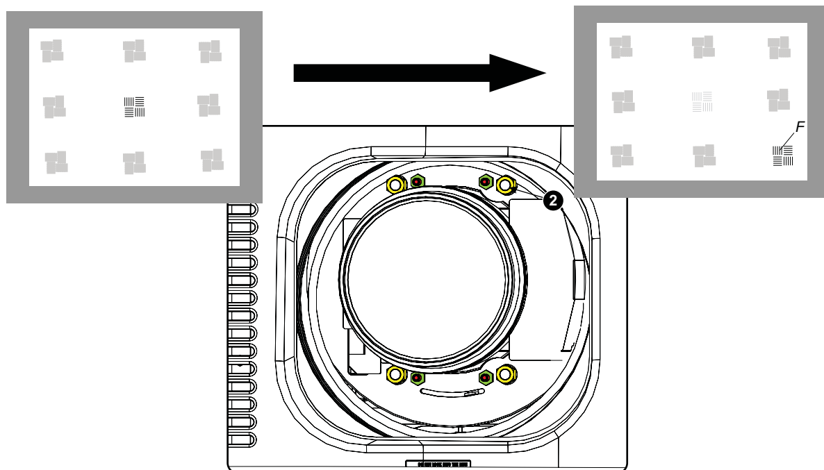
Изображение 3-39 Фокусировка в правом нижнем углу
