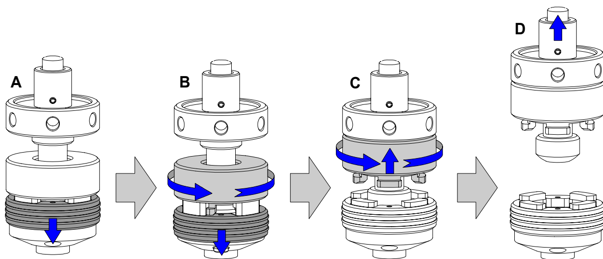
Изображение Е-5 Открывание фиксирующего адаптера
