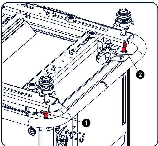
Изображение 3-47 Вставка болтов
