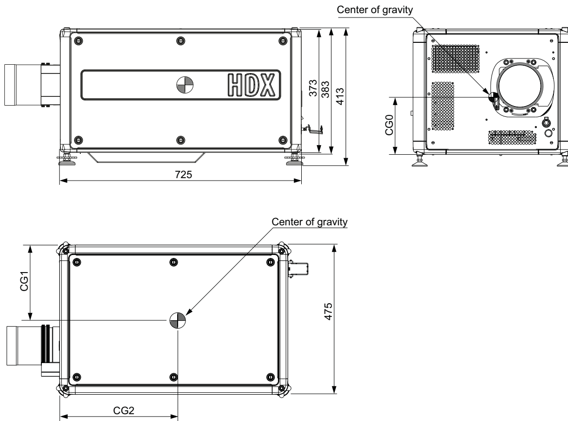
Изображение A-1 Размеры, мм
