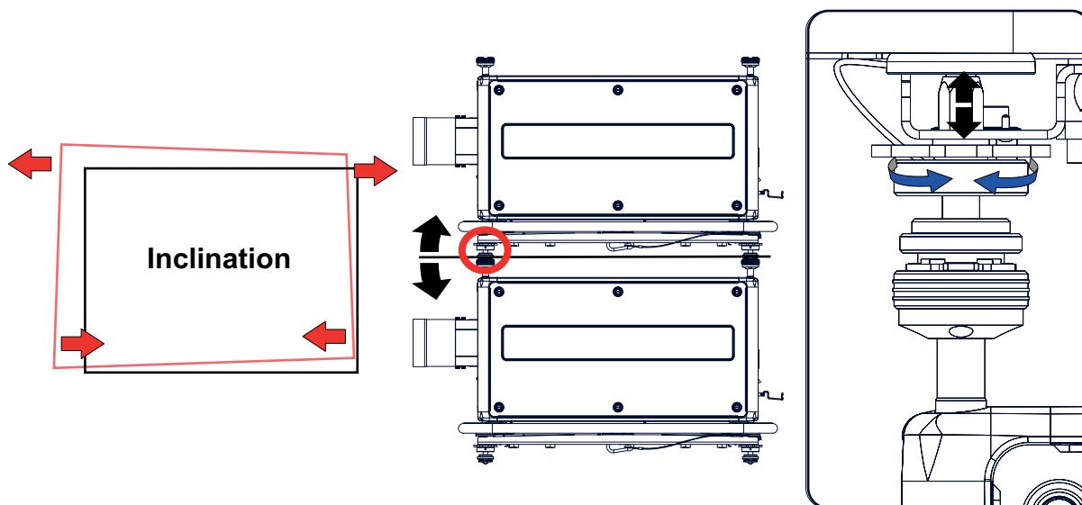
Изображение Е-7 Наклон изображений, проецируемых установленными друг на друга проекторами
