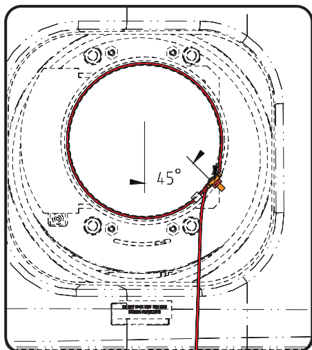
Изображение 3-30 Положение зажима
