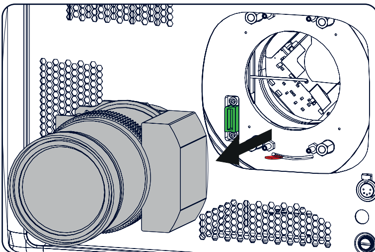
Изображение 3-28 Извлечение объектива
