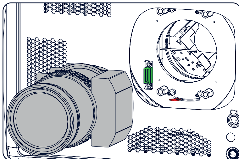
Изображение 3-25 Вставка объектива
