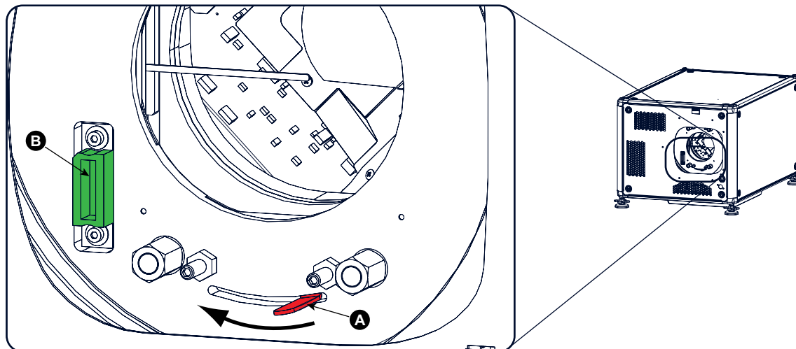
Изображение 3-24 Установка объектива, подготовка
