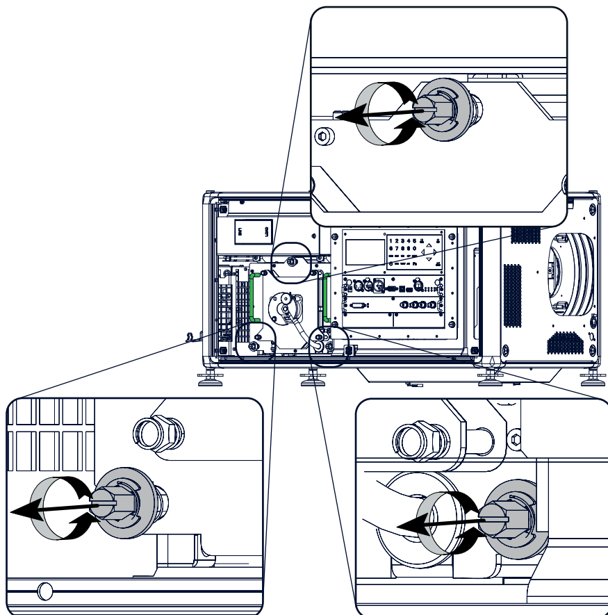
Изображение 16-3 Корпус лампы, невыпадающие винты
