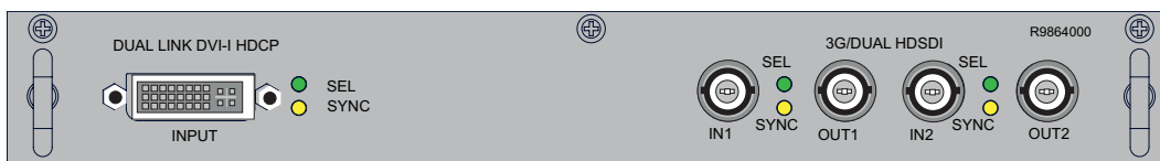
Изображение 4-2 Входы Dual Link DVI и 3G/Dual HDSDI (двухканальные)
