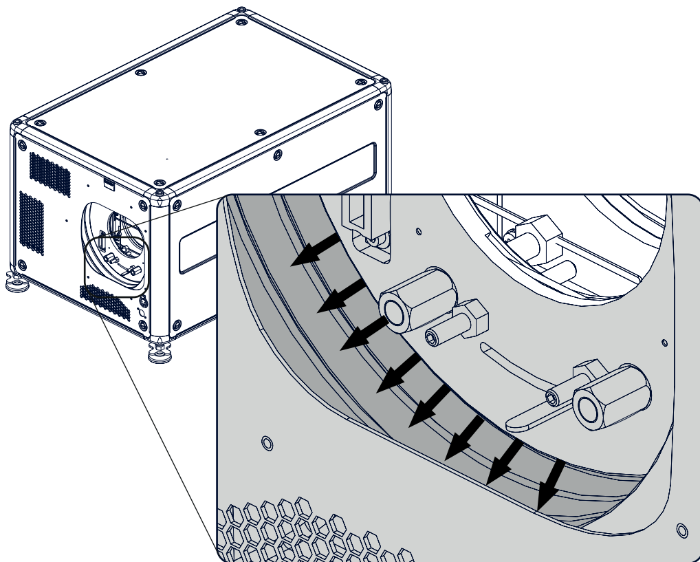
Изображение 16-6 Снятие пылезащитного кольца
