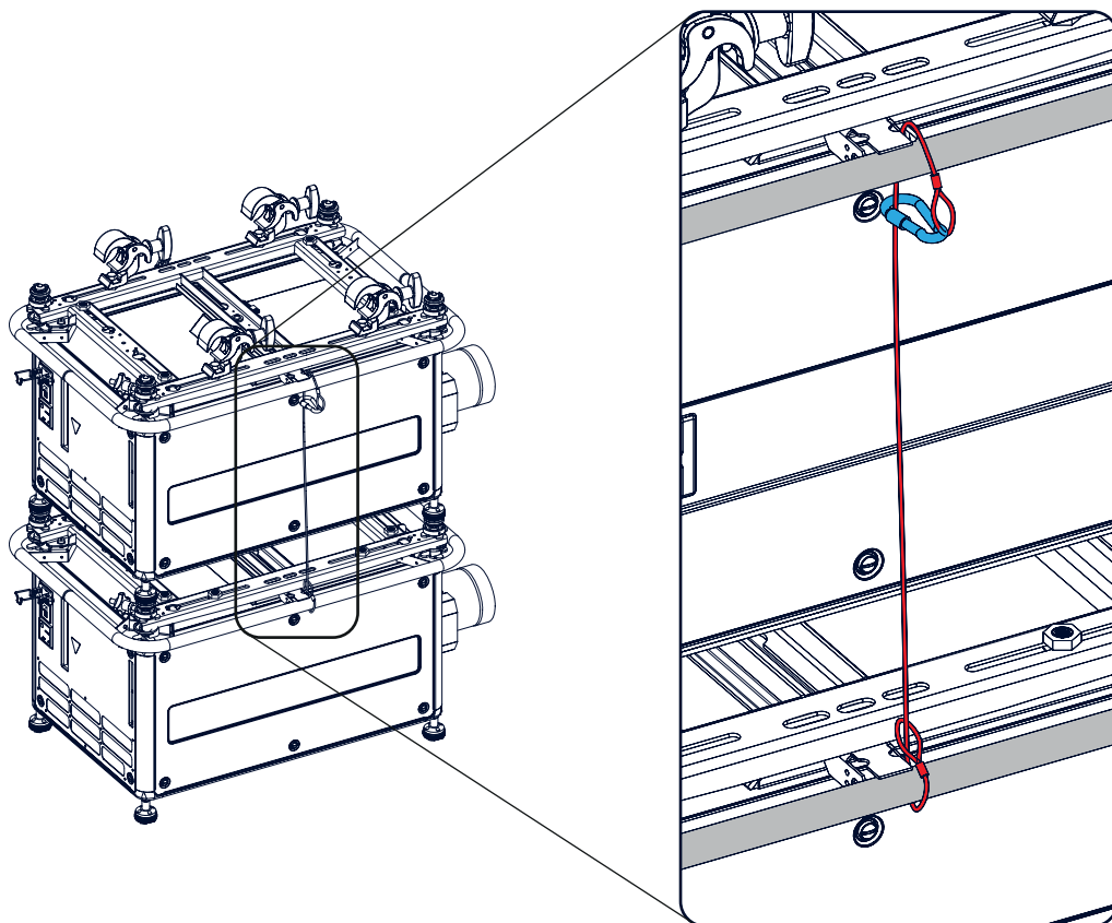
Изображение Е-4 Установка страховочных тросов
