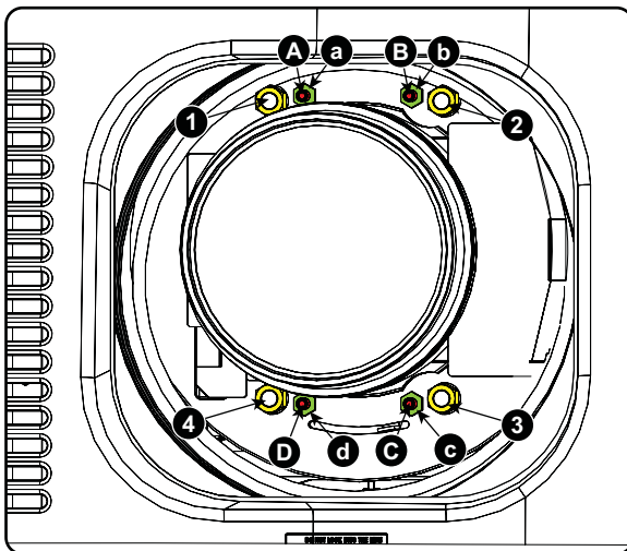
Изображение 3-35 Регулировка линии Шаймпфлюга
