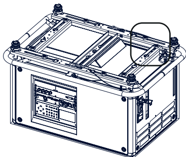
Изображение 3-49 Подвесные втулки
