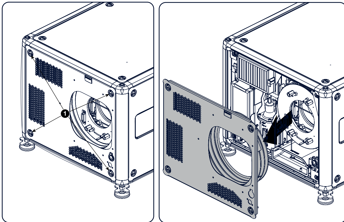
Изображение 16-7 Снятие передней крышки
