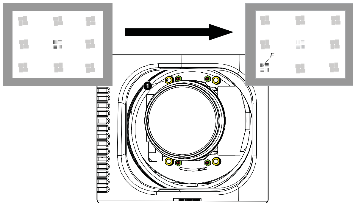
Изображение 3-38 Фокусировка в левом нижнем углу
