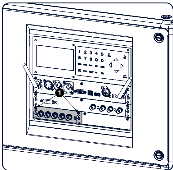
Изображение 16-2 Фиксация входа
