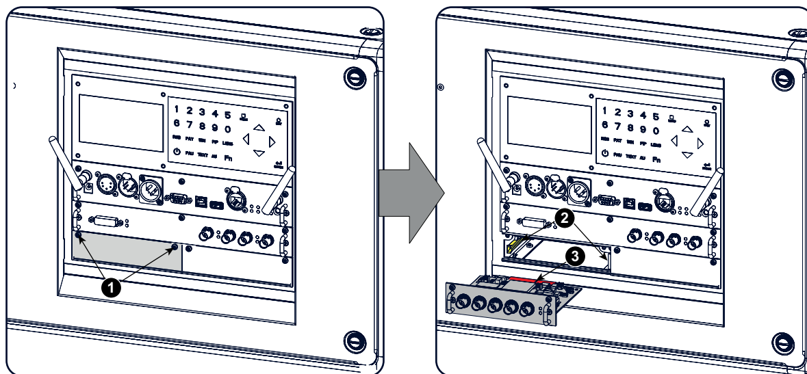
Изображение 16-1 Вставка входного модуля
