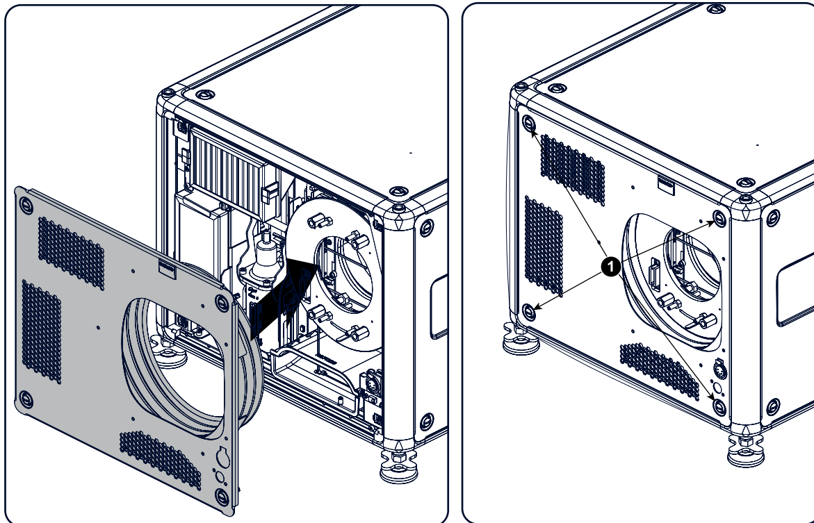
Изображение 16-8 Установка передней крышки
