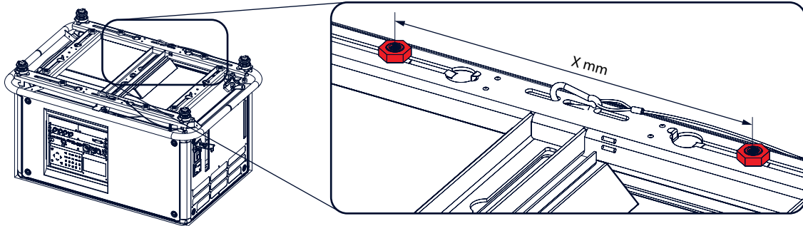
Изображение 3-51 Расстояние между подвесными втулками
