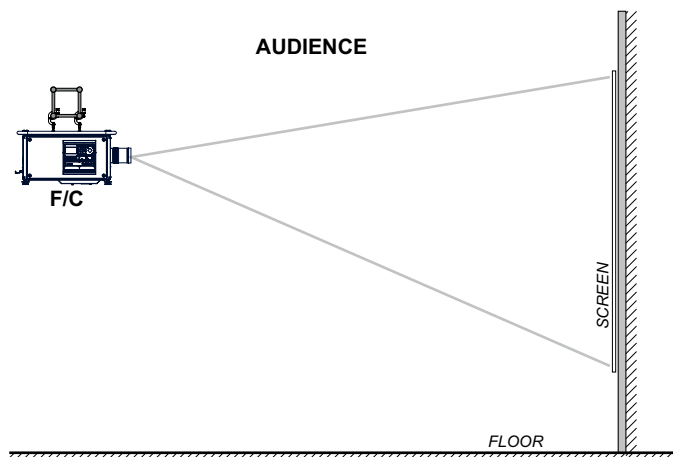
Изображение 2-5 Проецирование на светоотражающий экран, монтаж на потолке в нормальном положении
