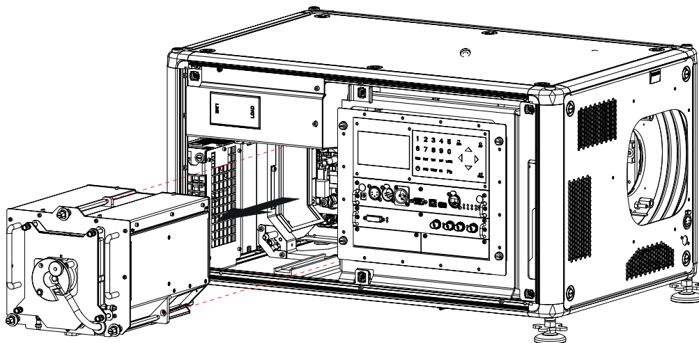
Изображение 16-4 Корпус лампы, извлечение
