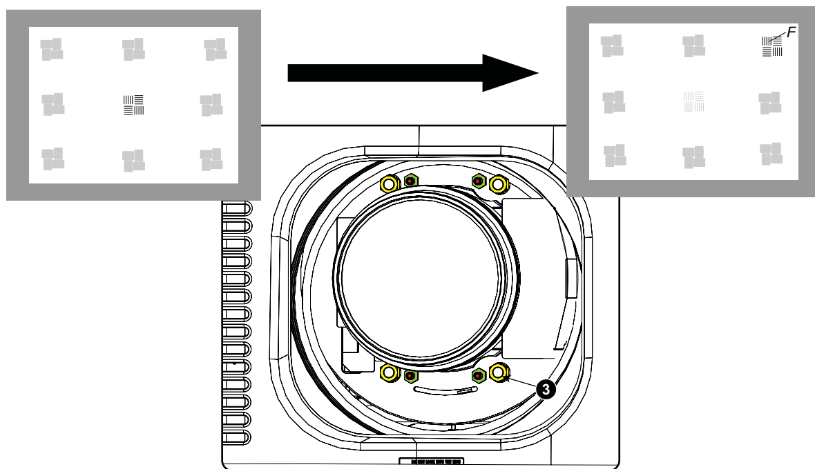
Изображение 3-40 Фокусировка в углу
