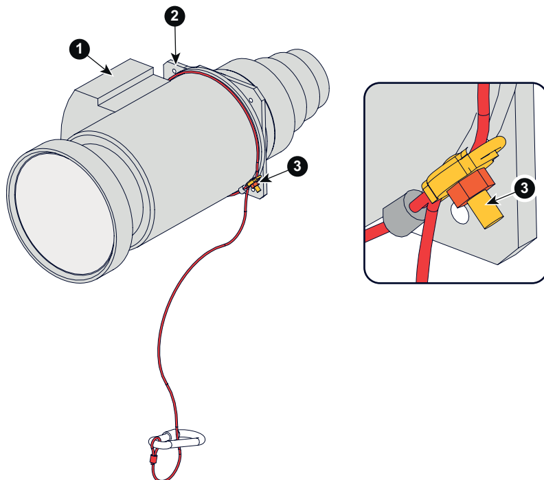
Изображение 3-29 Страховочный трос объектива
