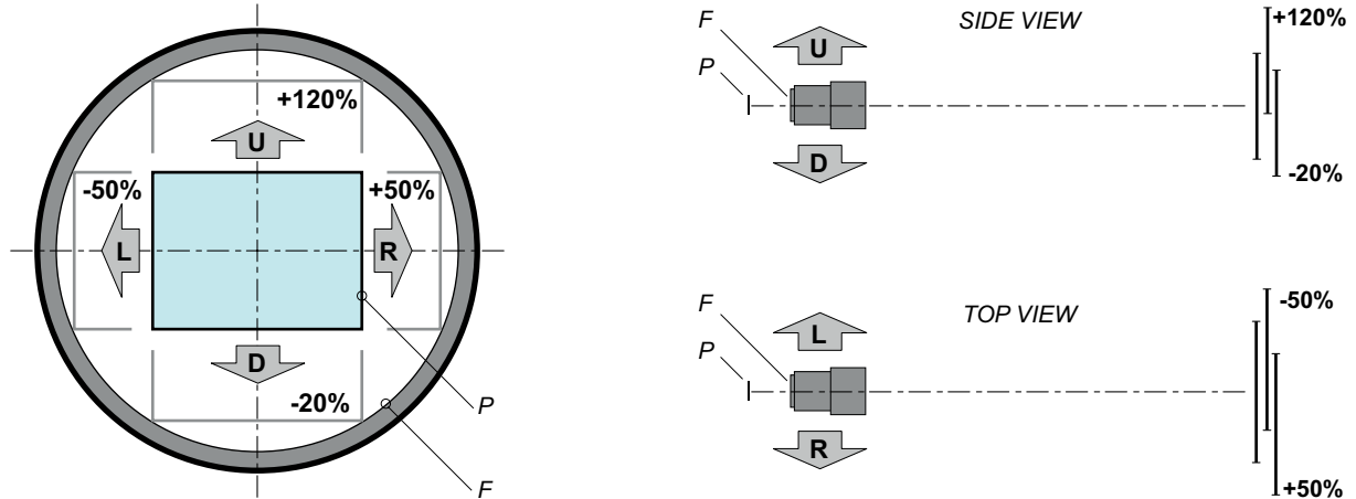
Изображение 2-9 Диапазон смещения по вертикали и горизонтали
