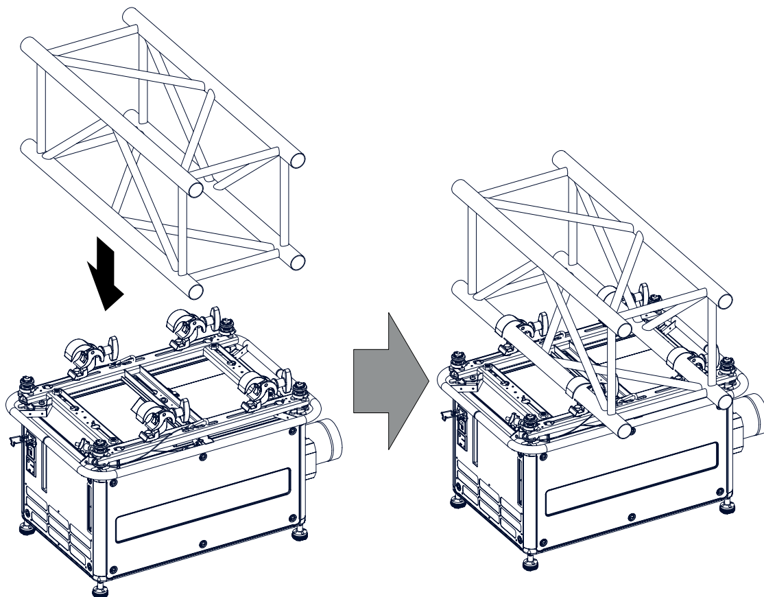
Изображение 3-53 Установка проектора на ферму
