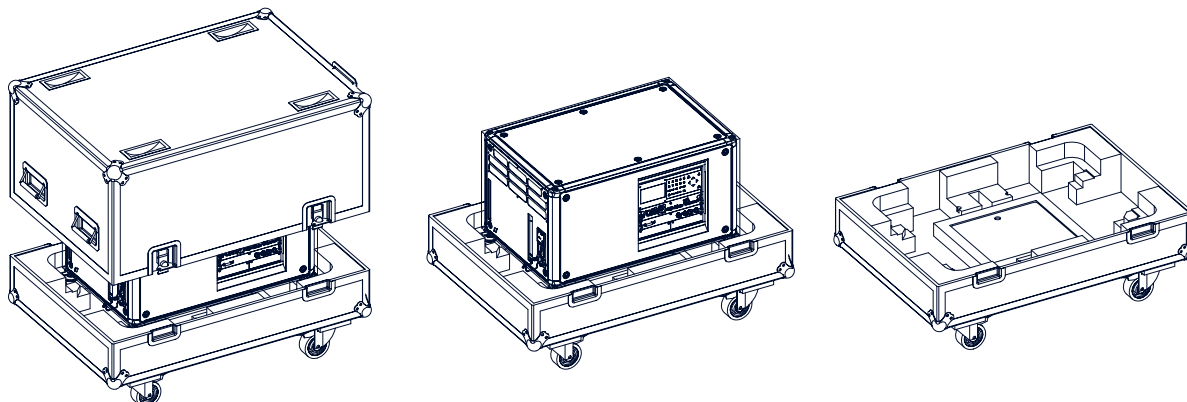
Изображение 2-3 HDX транспортный контейнер
