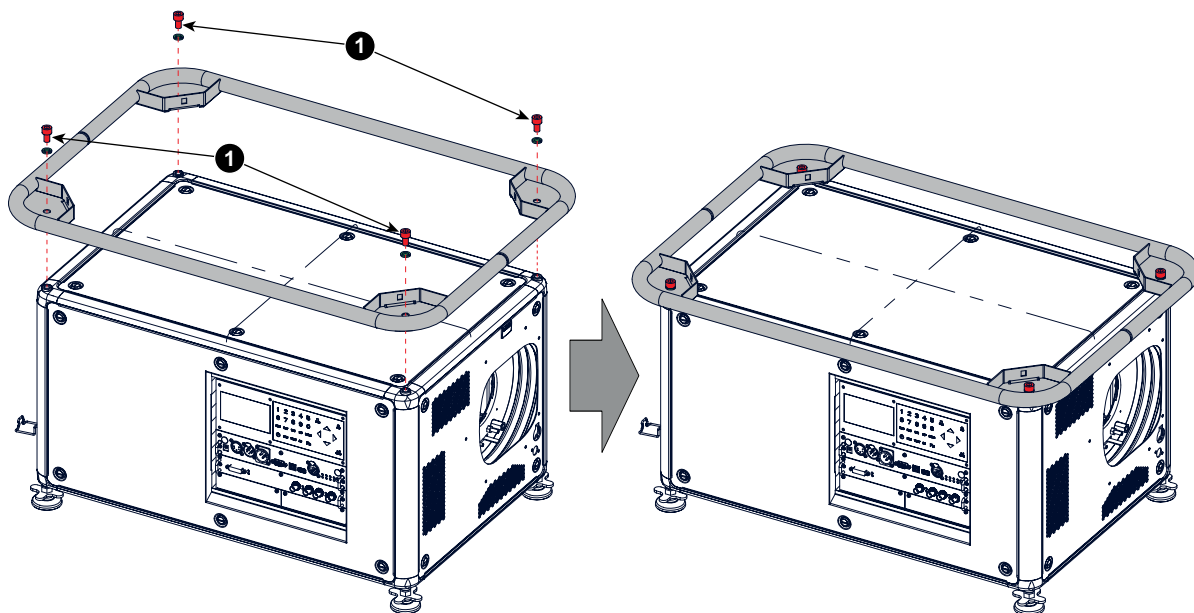
Изображение 3-48 верхняя рукоятка для переноски
