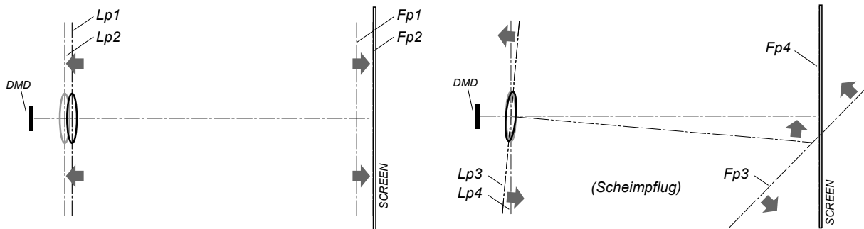
Изображение 3-34 Принцип Шаймпфлюга
