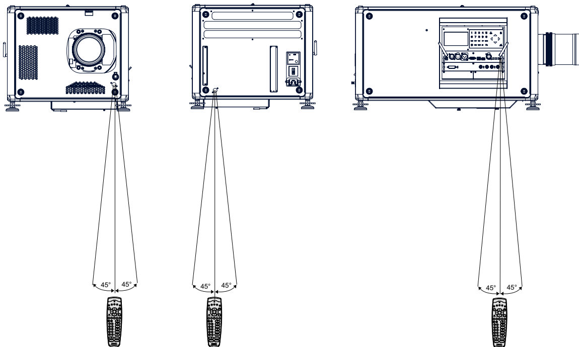
Изображение 5-8 Наведение пульта дистанционного управления на один из ИК-датчиков
