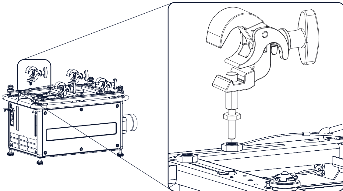
Изображение 3-52 Установка подвесных зажимов
