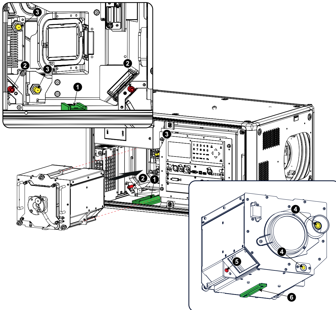
Изображение 16-5 Вставка корпуса лампы
