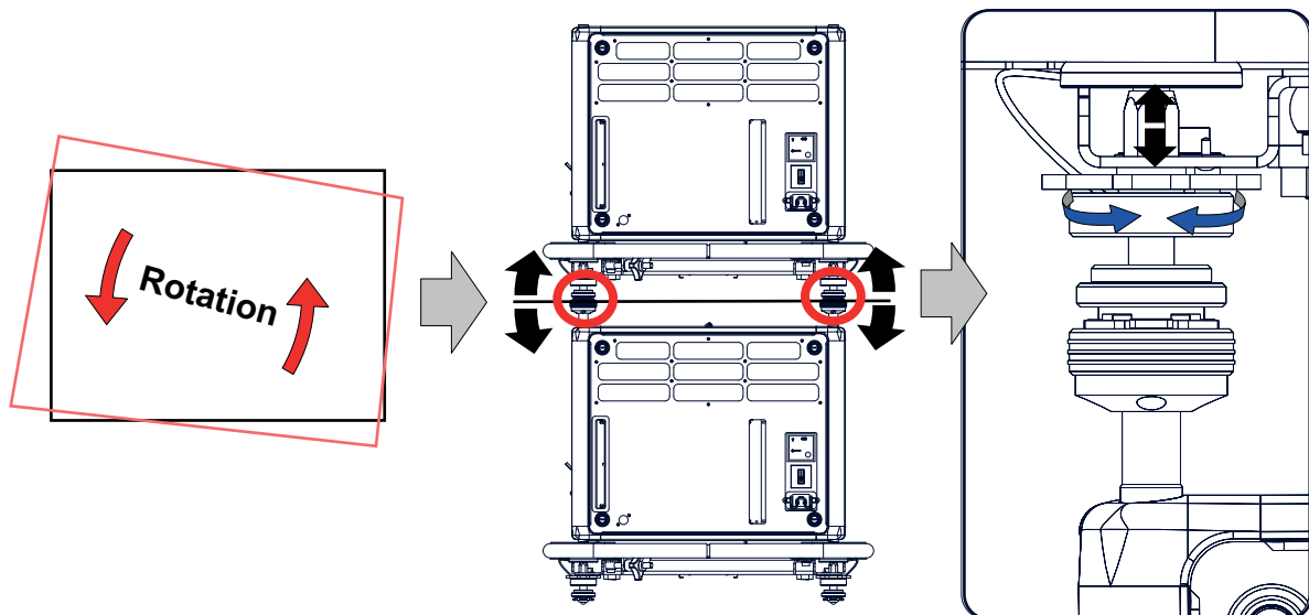
Изображение Е-6 Поворот изображений, проецируемых установленными друг на друга проекторами
