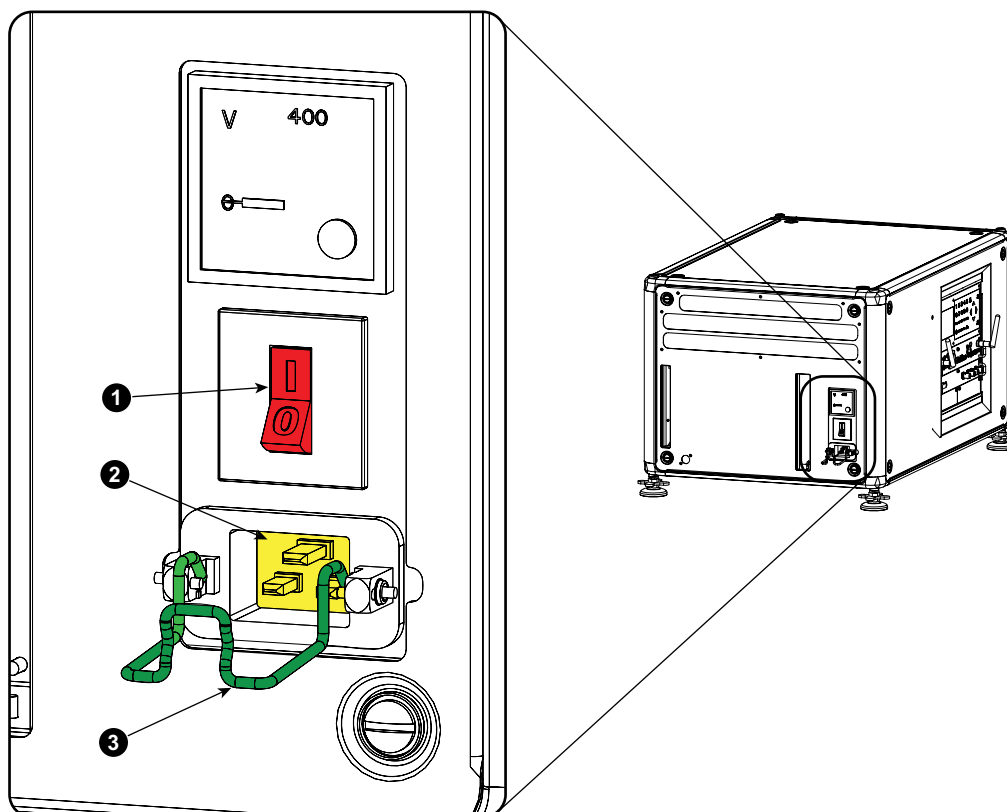
Изображение 3-42 Вход питания
