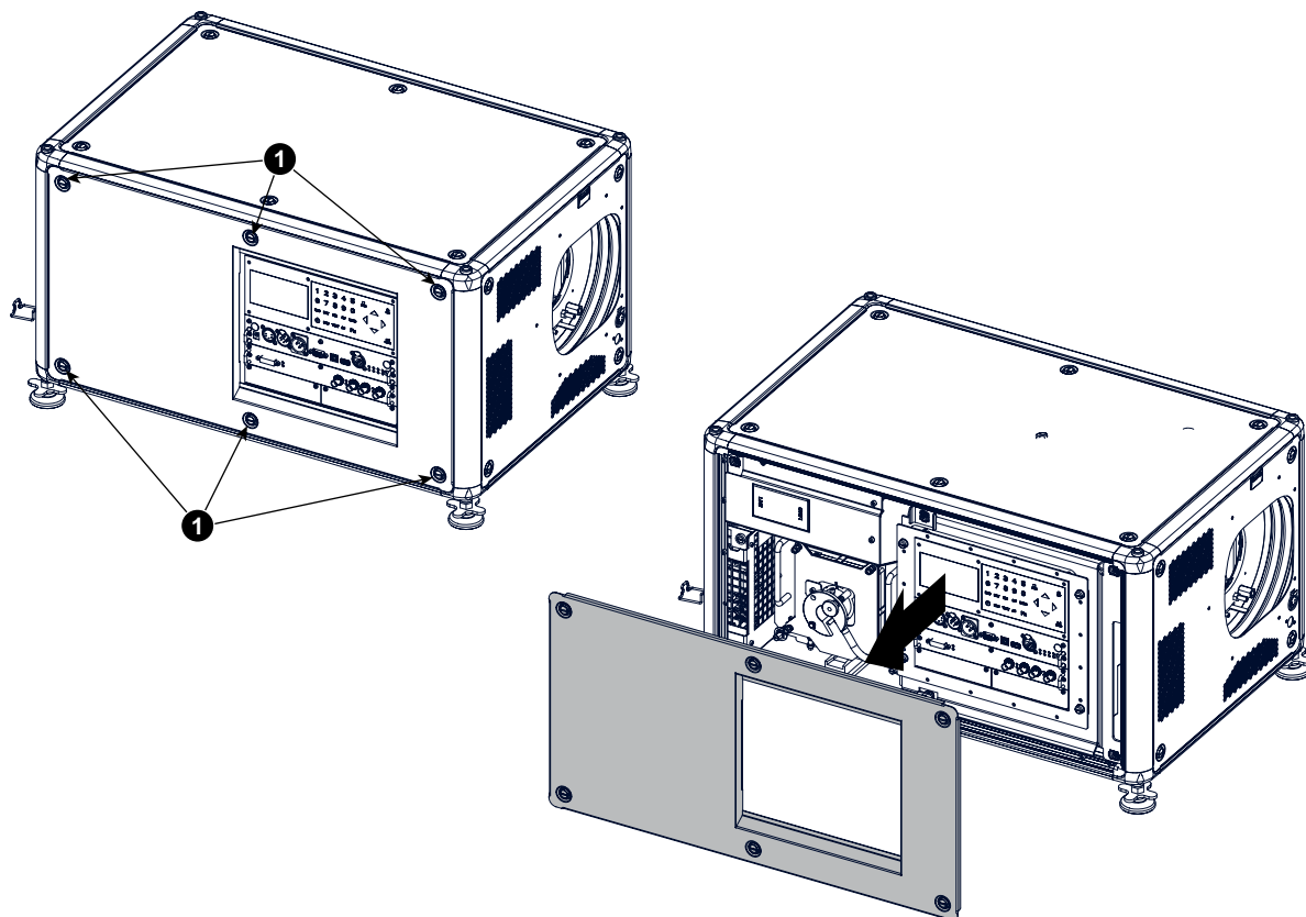
Изображение 16-10 Боковая крышка лампы
