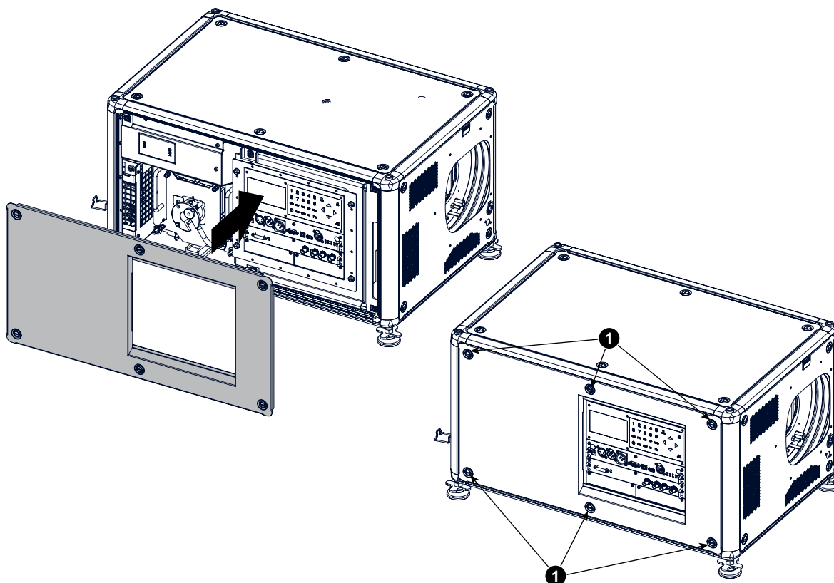
Изображение 16-11 Боковая крышка лампы
