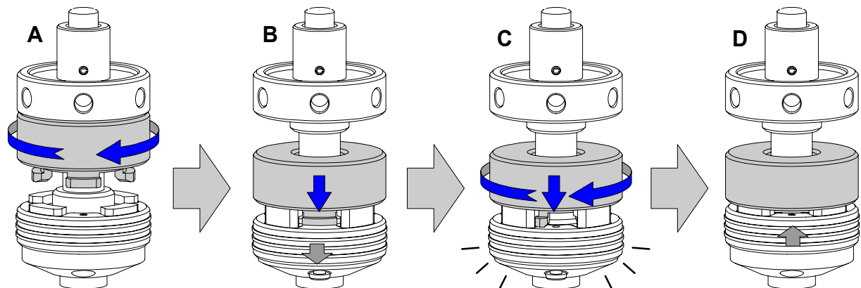
Изображение Е-3 Закрывание фиксирующих адаптеров
