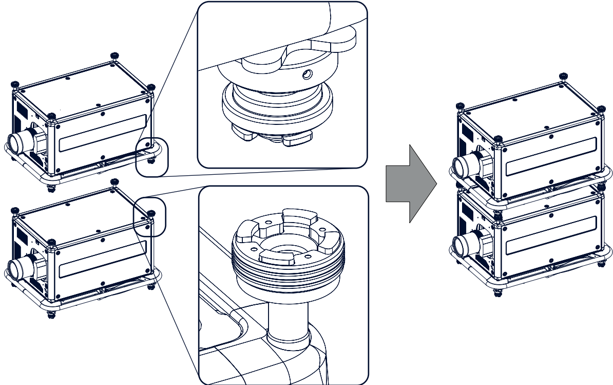
Изображение Е-2 Конфигурация из двух проекторов
