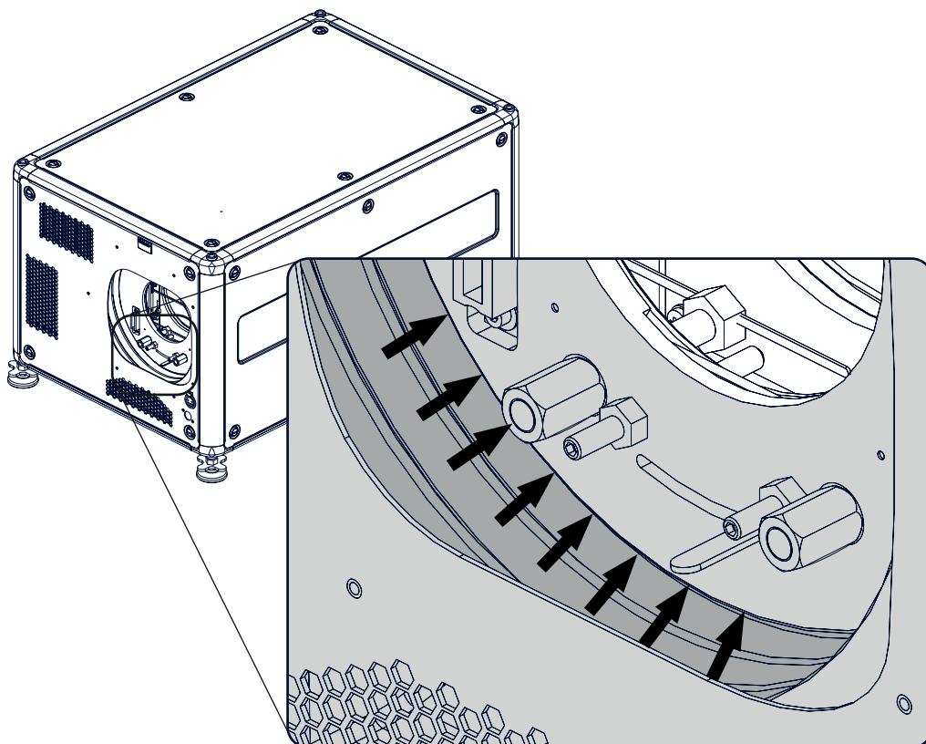
Изображение 16-9 Установка пылезащитного кольца
