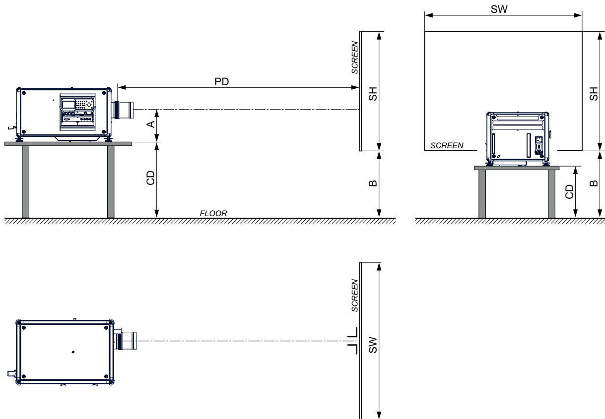
Изображение 2-8 Размещение проектора
