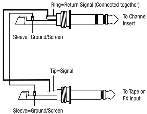
Signalabgriff: Direktausgang (Ermöglicht die Nutzung des Insert-Punkts als Direktausgang, ohne Unterbrechung des eigentlichen Signalflosses.)
