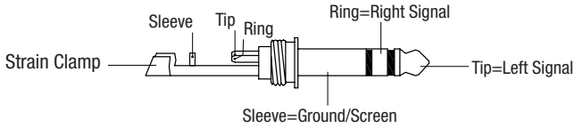
Anschluss: Kopfhörer, Stereo-Return 6,3-mm-Stereoklinke (TRS)
