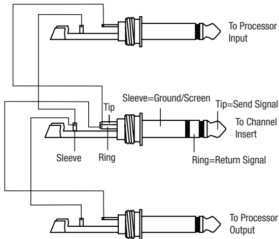
„Y“-Stereokabel für Insert-Verbindungen (Erforderlich, wenn der externe Signalprozessor getrennte Buchsen für Ein- und Ausgangssignale besitzt.)
