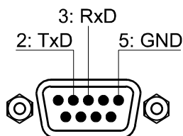
Illustration 4.9: Câblage de l'Interface RS-232
