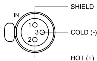
Abbildung 4.5: Belegung AES/EBU-IN
