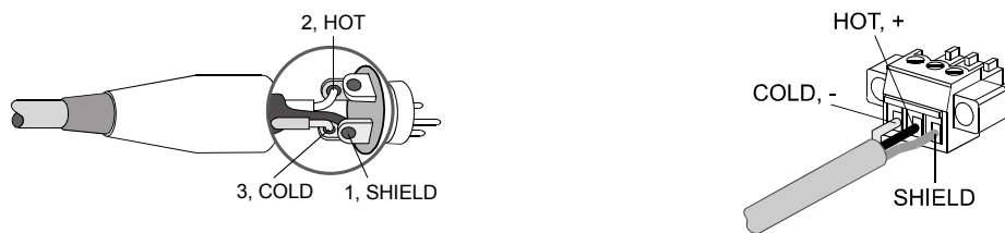
Abbildung 2.10: Symmetrische Beschaltung des Eingangs
