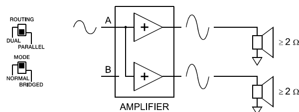
Abbildung 2.8: Einspeisung an Eingang A bei Betriebsart PARALLELE
