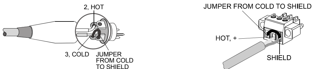
Abbildung 2.11: Unsymmetrische Beschaltung des Eingangs
