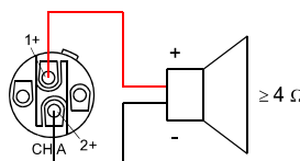
Abbildung 2.16: Lautsprecheranschluss in Betriebsart BRIDGED an Speakon A
