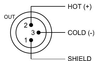
Abbildung 4.6: Belegung AES/EBU-OUT
