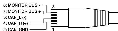
Illustration 4.8: Câblage de la prise CAN
