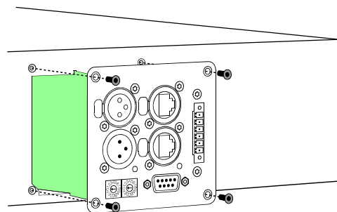
Abbildung 4.1: Einbau des RCM-26 in eine Endstufe
