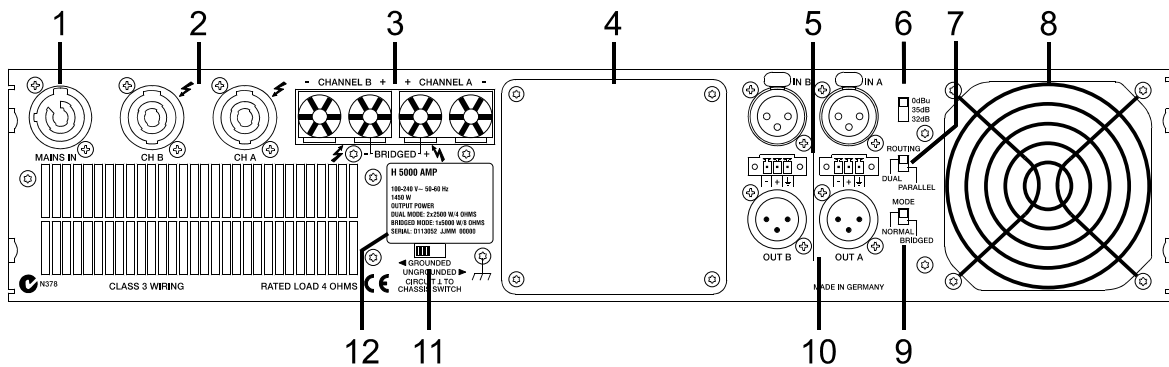
Abbildung 2.2: H2500/H5000 Rückseite
