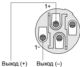
а) для поканального подключения
