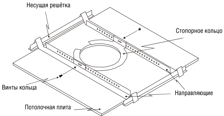
Рис. 4. Установка потолочного громкоговорителя закрытого типа Yarden 4-C
