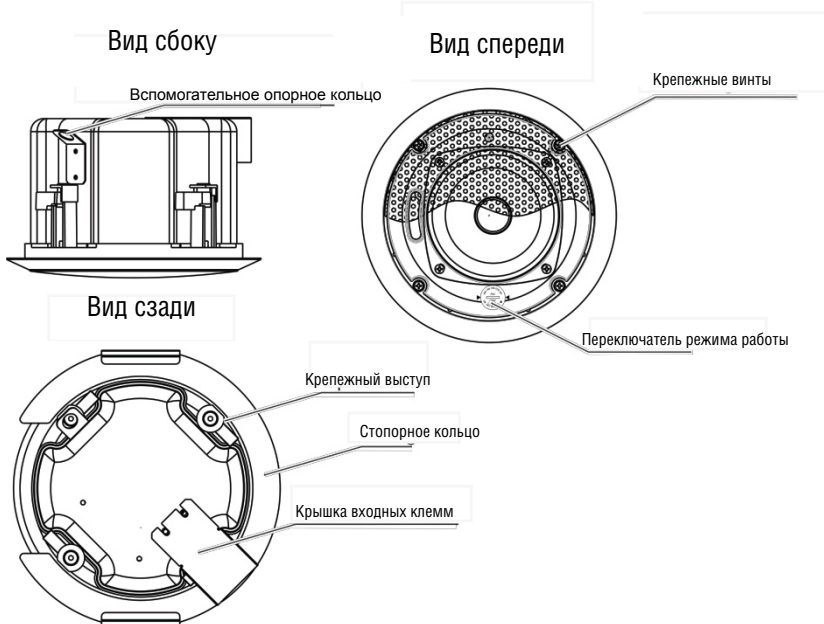
Рис. 2. Потолочный громкоговоритель закрытого типа Yarden 4-C
