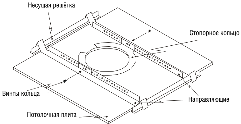
Рис. 4. Установка потолочного громкоговорителя закрытого типа Yarden 6-CH
