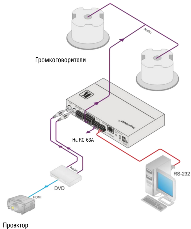
Рис. 1. Установка потолочного громкоговорителя закрытого типа Yarden 6-CN в зале заседаний
