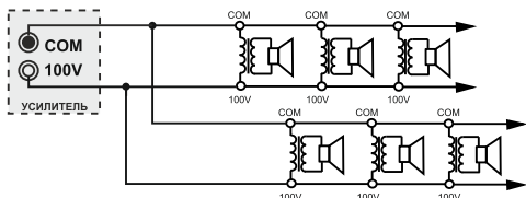
параллельное соединение:
